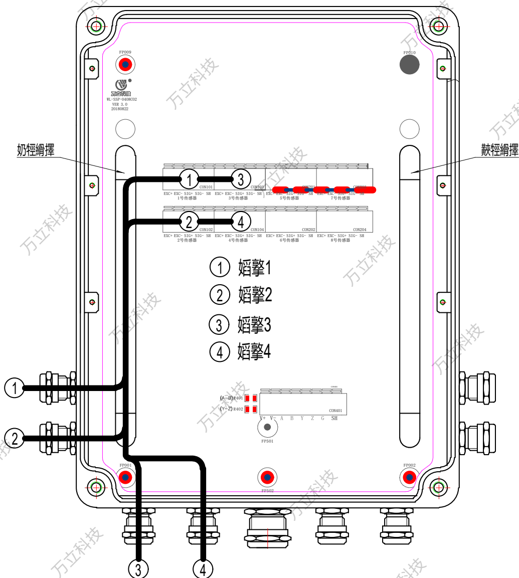
图 3-4 ZCS-30-WB 弯板式动态汽车衡的称重传感器接线
