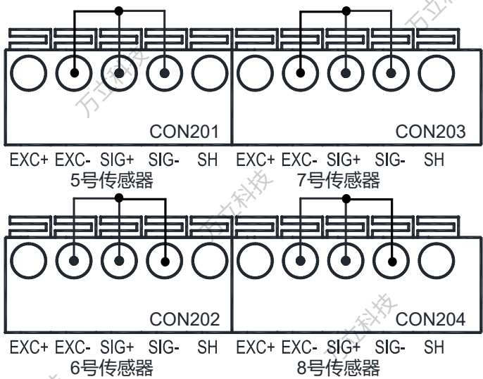
图 3-3 剩余通道的处理方法
