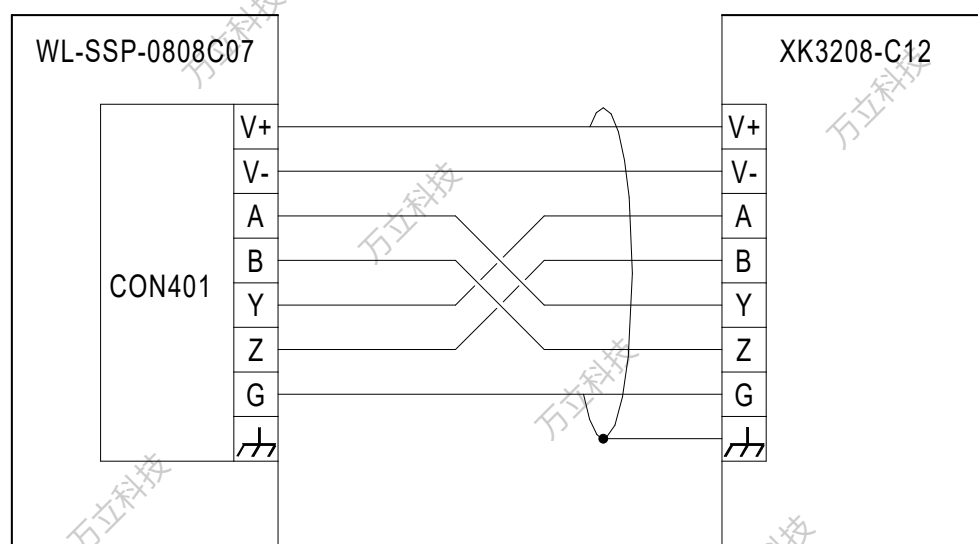
图 3-5 C07 处理器与称重仪表的接线
